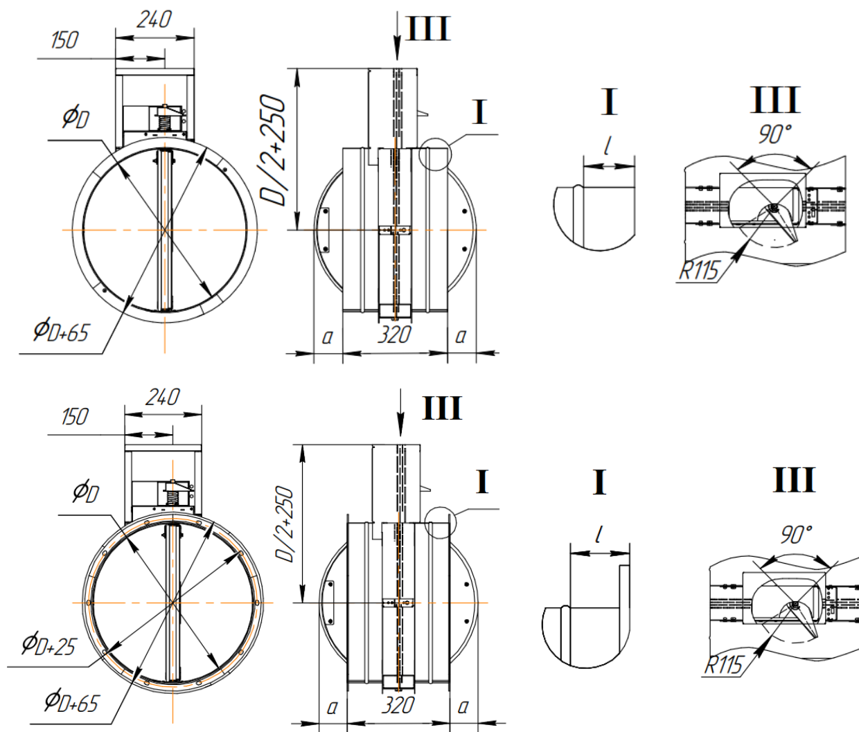
Рисунок 2 – Клапаны KPNO с приводом ЕМ, 500 \leq D \leq 1000
