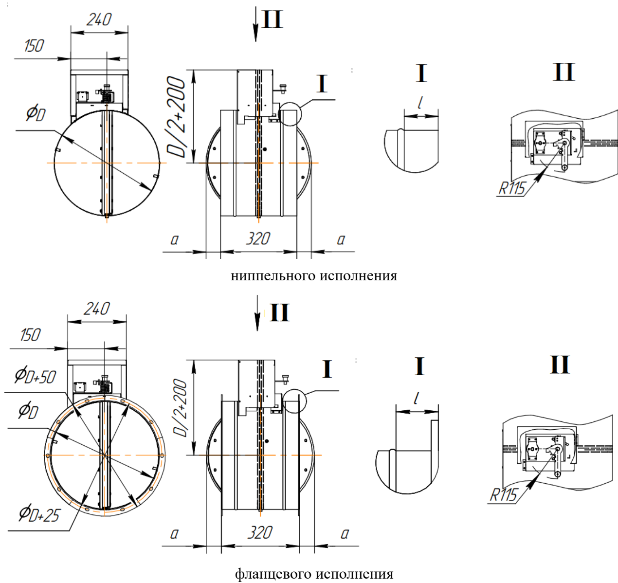
Рисунок 1 – Клапаны KPNO с приводом EM, D \leq 450
